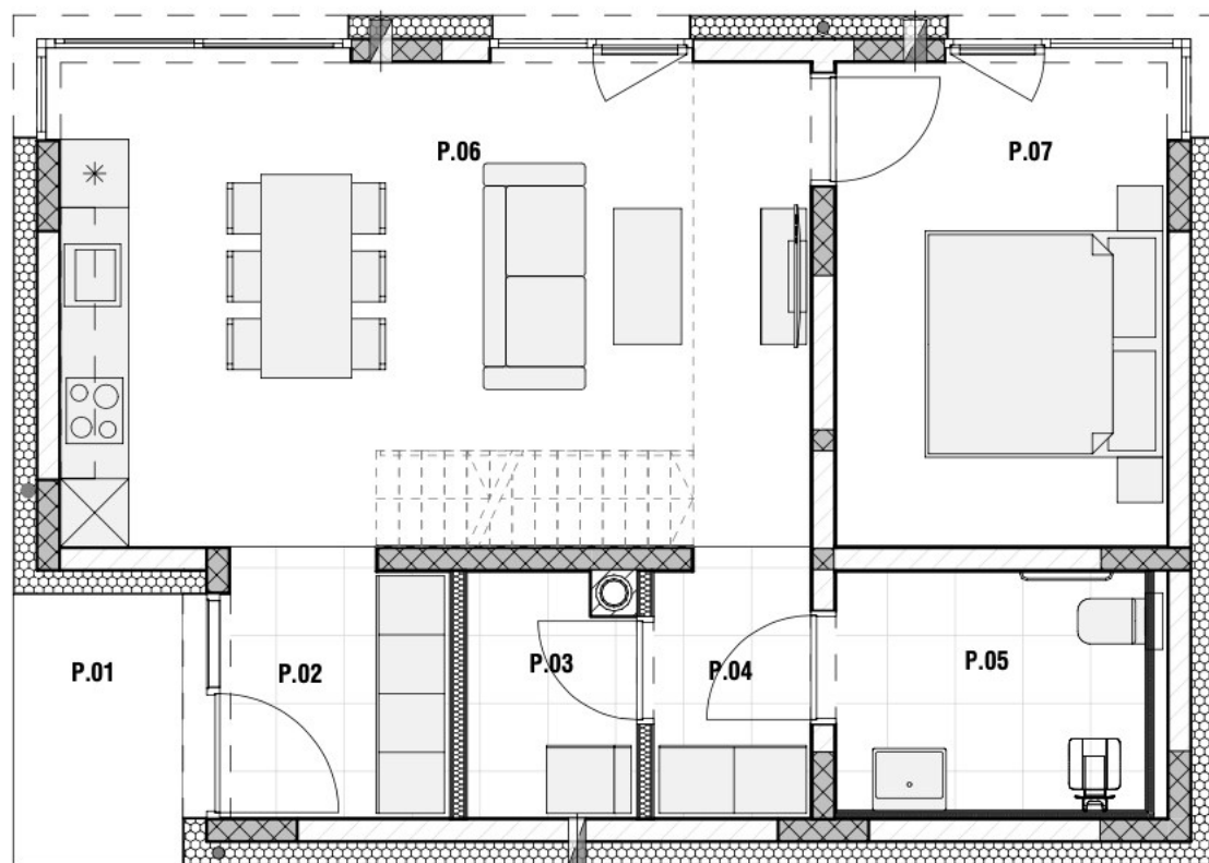
TLORIS PRITLIČJA
