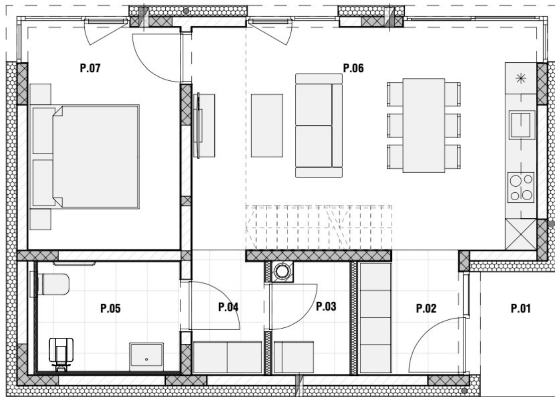
TLORIS PRITLIČJA
