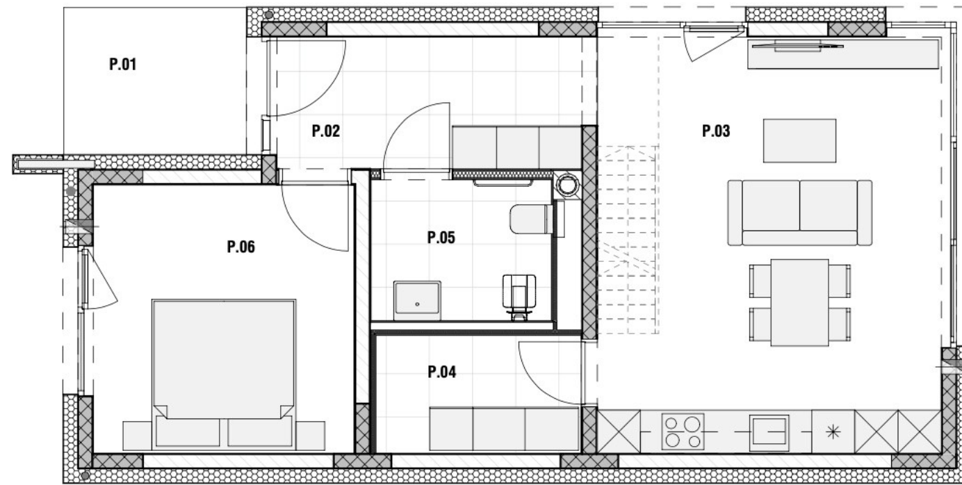
TLORIS PRITLIČJA
