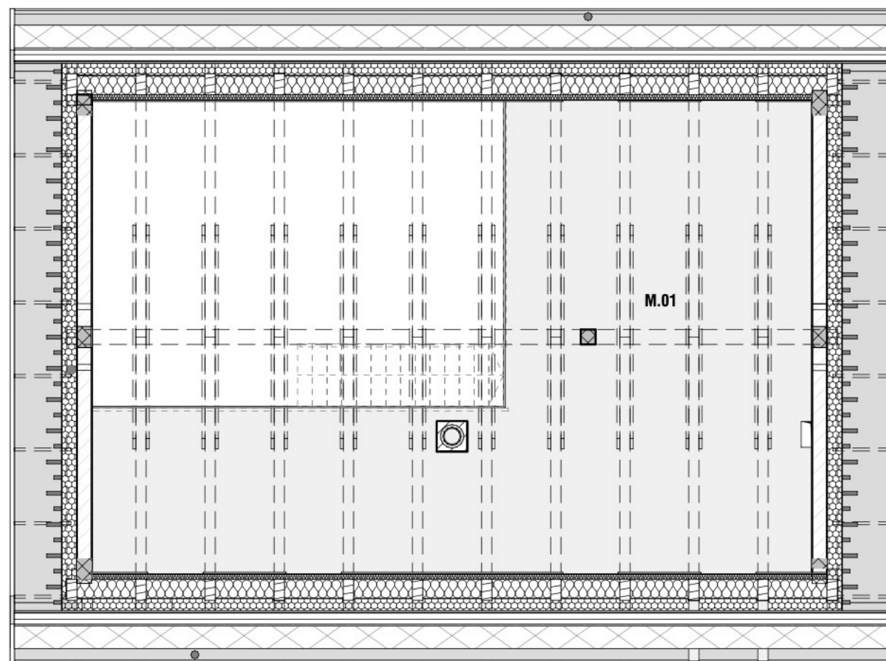
TLORIS MANSARDE
