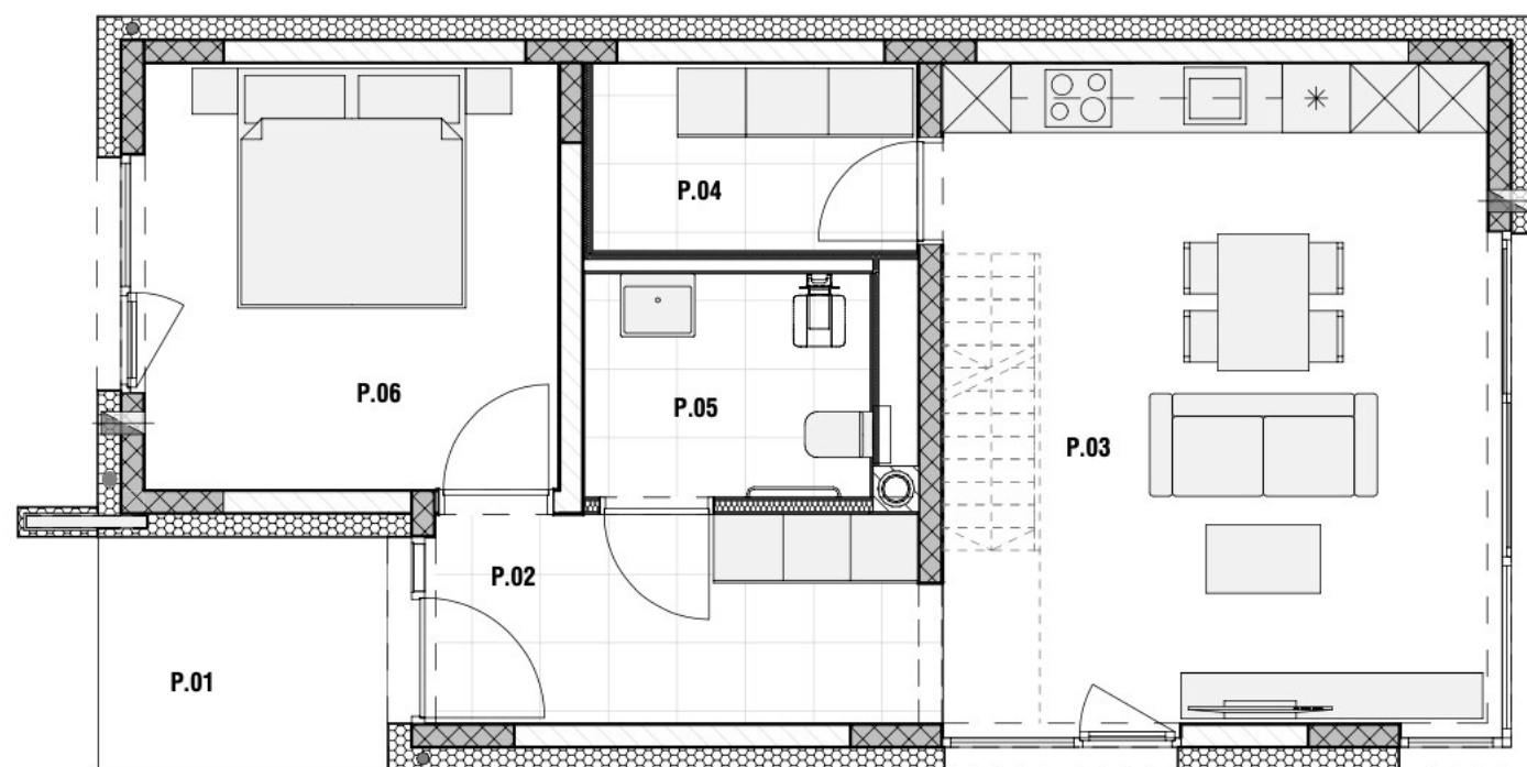
TLORIS PRITLIČJA
