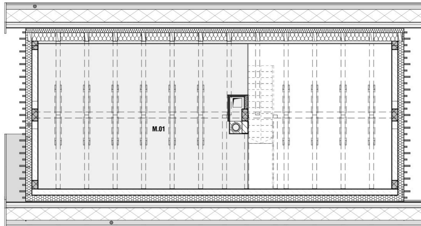
TLORIS MANSARDE
